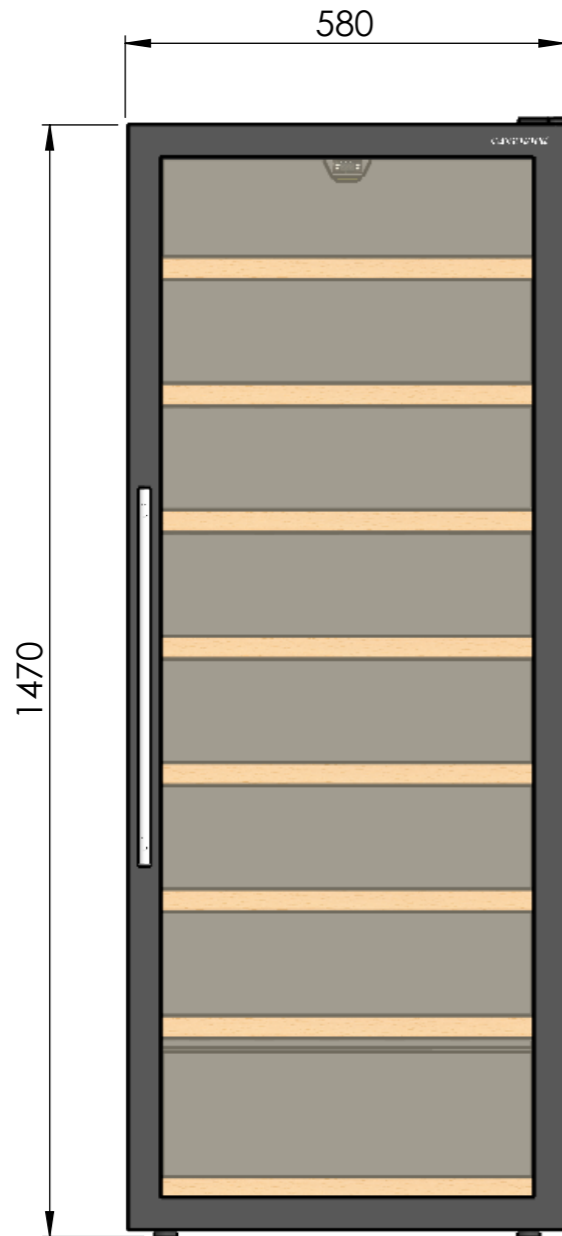
ALZADO
