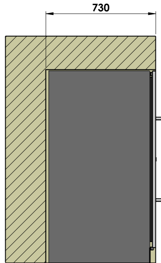
SECCIÓN B-B ESCALA 1 : 15
