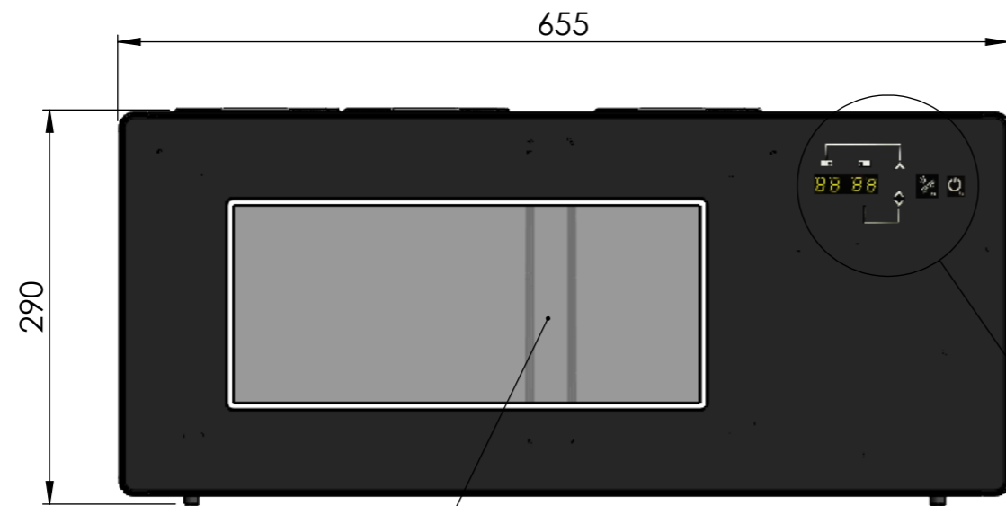
ALZADO
