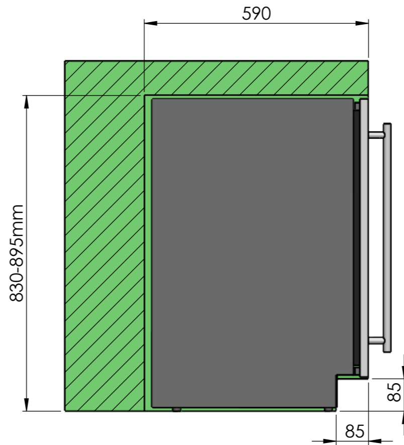
SECCIÓN I-I ESCALA 1 : 10
